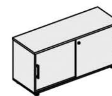
9622 103x46x58 двери купе с замком
